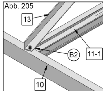
Abb. 204 bis 207: Ausführung mit Grundschiene (Standard)
