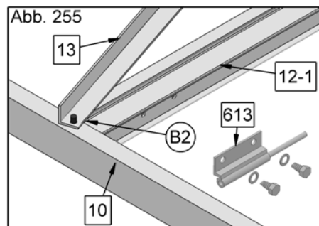
Abb. 254 bis 257: Ausführung mit Grundschiene (Standard)
