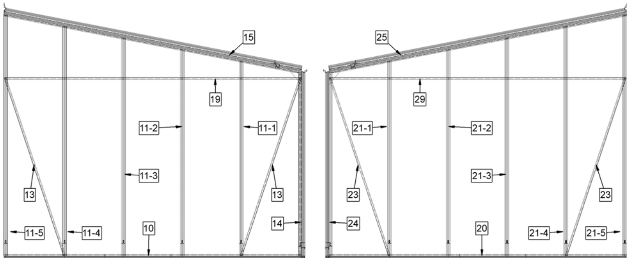
Giebel „Links“
