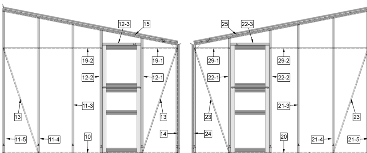
Türgiebel „Links“
