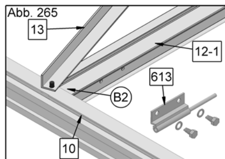
Abb. 264 bis 267: Ausführung mit optionalem Basisrahmen
