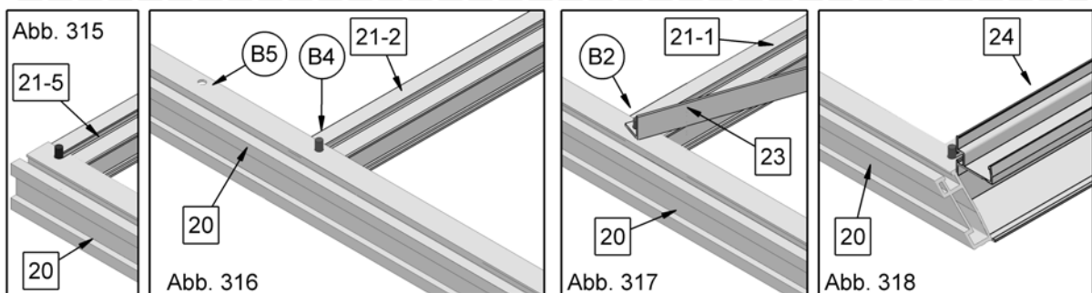
Abb. 315 bis 318: Ausführung mit optionalem Basisrahmen
