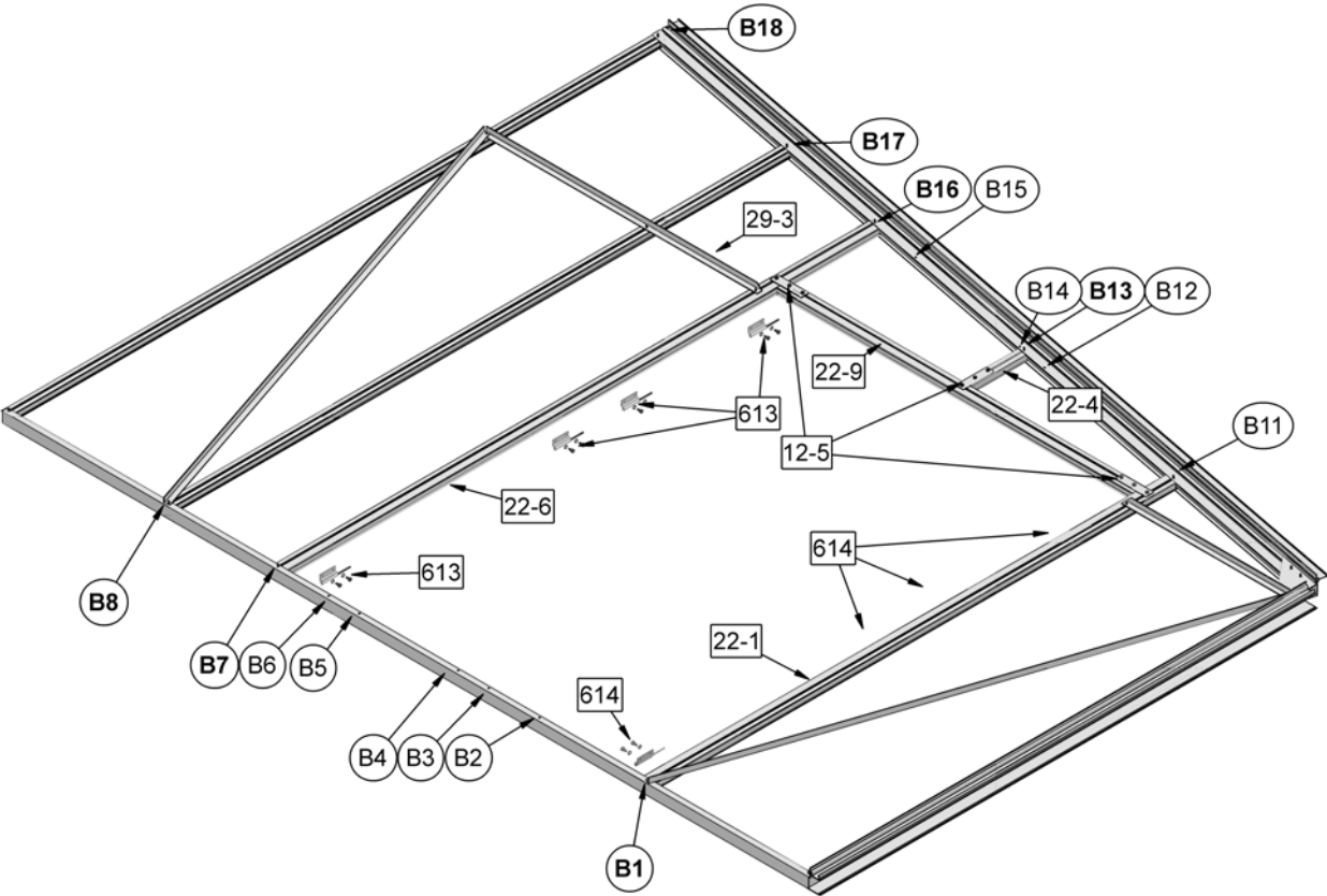
Abb. 375
