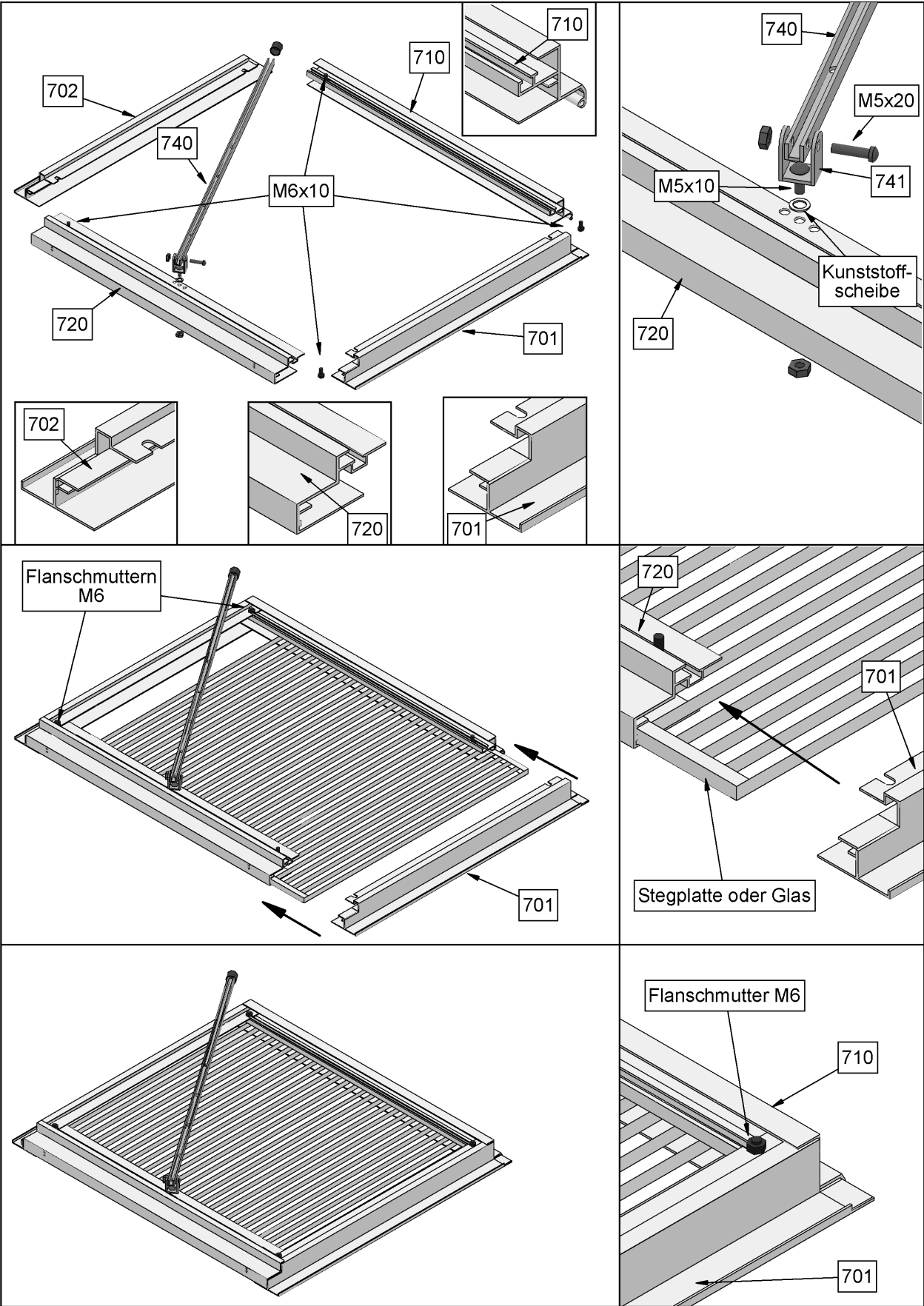
Abb. 450
