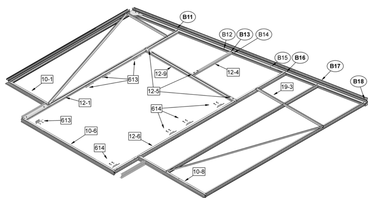
Abb. 276
