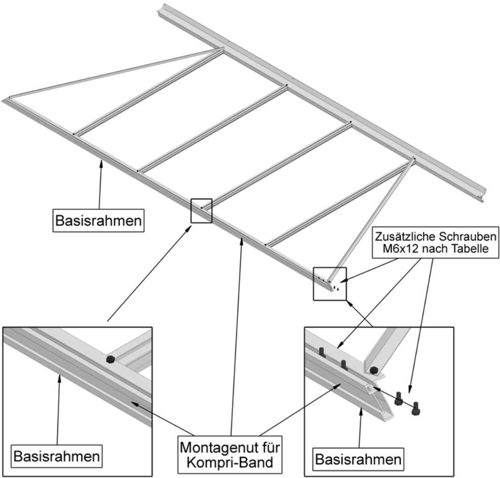
Abb. 490
