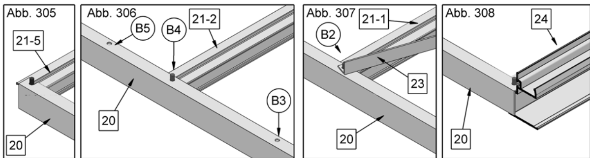
Abb. 305 bis 308: Ausführung mit Grundschiene (Standard)
