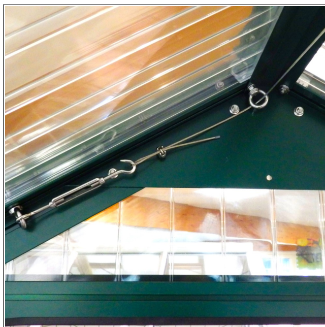
Abb. 2 (F. Drahtseil fixieren und spannen)
