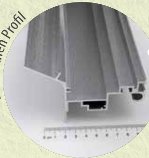
T-Profil Seitenwand und Dach
